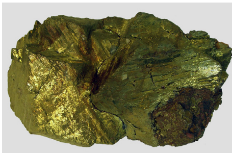
Халькопирит
